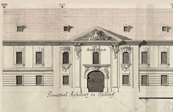
Časť inžinierskeho plánu prestavby arcibiskupského kaštieľa v Podunajských Biskupiciach z rokov 1779/80. Na základe odborných nákresov predpokladáme, že Melchior Hefeleg sa zúčastnil aj pri týchto stavbách.
