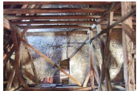
Neskorostredoveký atypický krov nad trojlodím kostola z konca 15. storočia.
